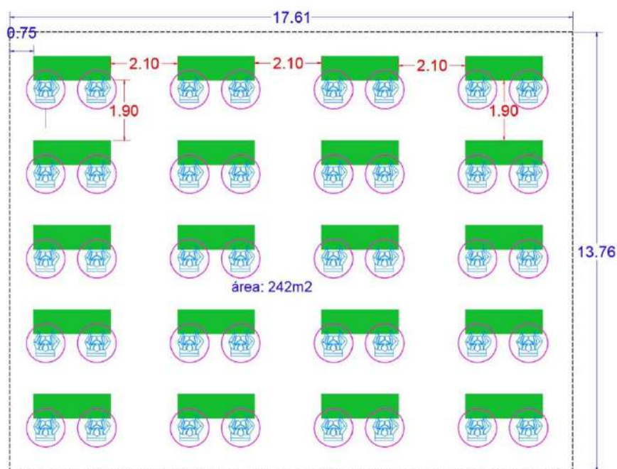
Esquema 6 Montaje escuela, con tablón (2.44 x 0.75 m) para 2 pax
