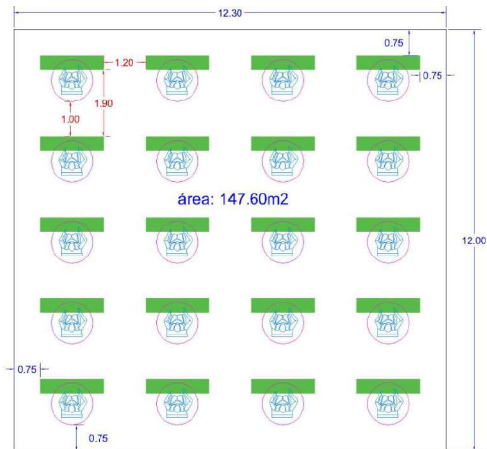
Esquema 1 Montaje escuela, con tablón (1.80 x 0.40 m)
