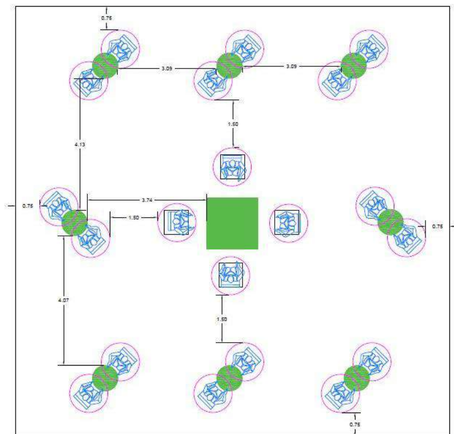
Esquema 31 Montaje tipo coctel social, mesa redonda y sala lounge
