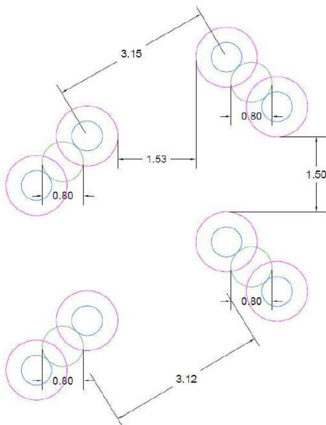
Esquema 30 Montaje tipo coctel social, mesa redonda
